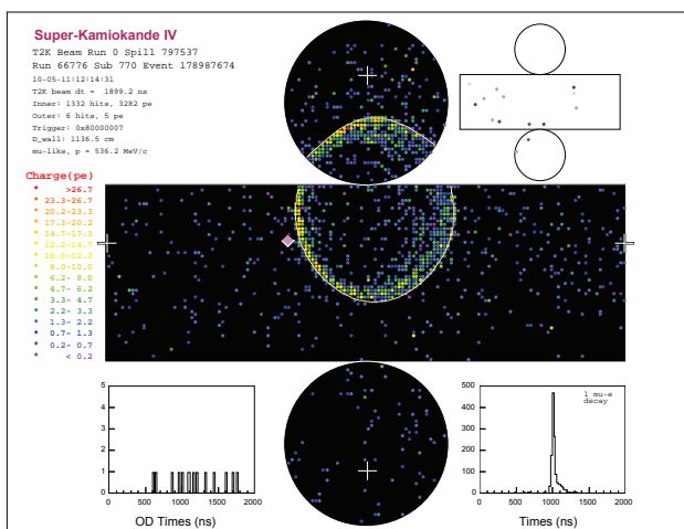
図 A.6 スーパーカミオカンデにおいて観測されたミューニュートリノイベントの候補の例
