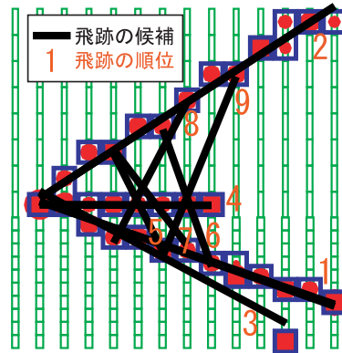
図 7.5 飛跡の候補を構成
