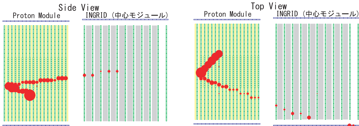
図 10.3 Proton Module におけるニュートリノ反応からの二次粒子が INGRID に入射したイベント
