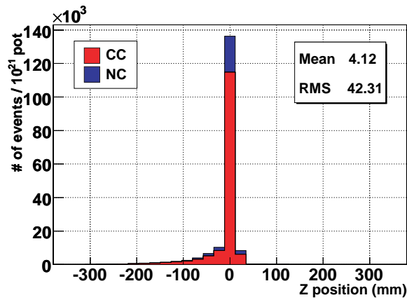
図 7.12 シミュレーションにより評価した、再構成された反応点 - 実際の反応点 (Z 座標) 1 ビンはトラッキングプレーン間の距離 (2.3cm)
