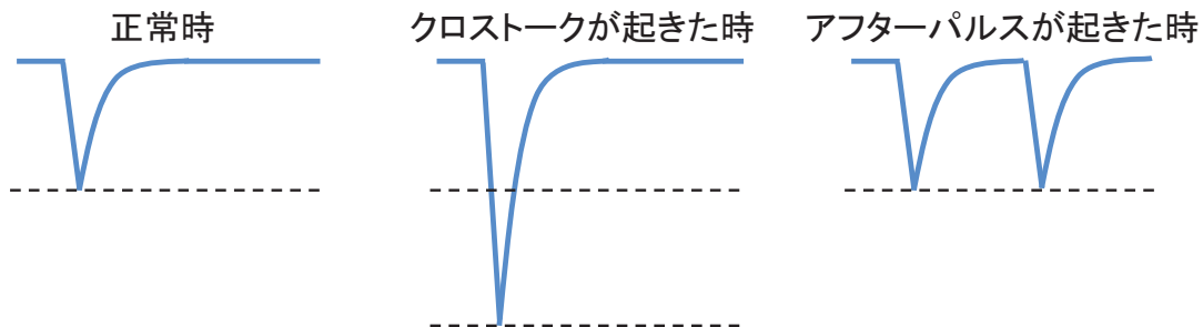
図 3.23 正常時とクロストーク、アフターパルスが起きたときの波形
