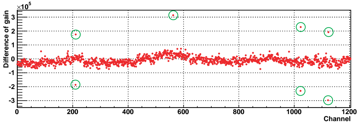
図 8.16 組立前と組立後のゲインの測定値の差 (緑色の丸で囲まれた点が差が激しいチャンネル)
