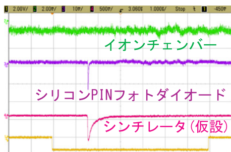
図 A.1 ミュオンモニターの初信号
