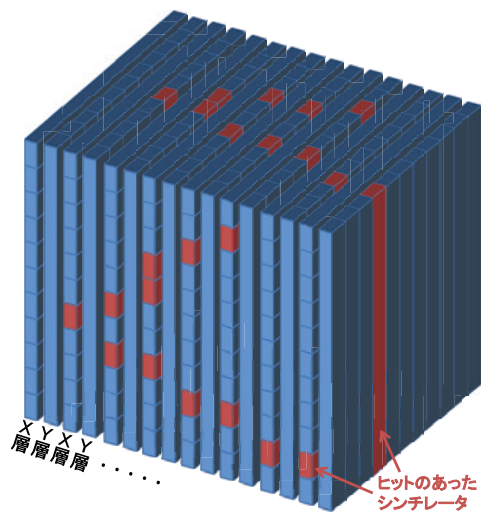
図 3.10 3次元飛跡の再構成
