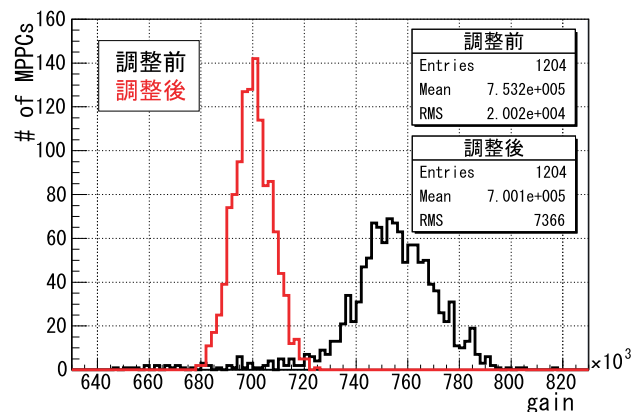
図 8.53 調整前と調整後の全 1204 チャンネルのゲイン
