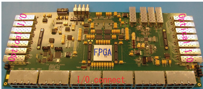
図 3.32 Back End Board (BEB)
