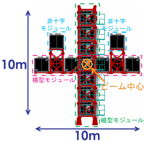
図 2.16 on-axis 検出器 INGRID ビーム中心には 2 台のモジュールが重なっている
