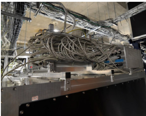
図 8.50 Proton Module のケーブル接続
