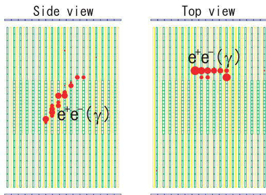
図 6.27 シミュレートされた壁での CC1\pi^0 反応で生成された \pi^0 の崩壊により生成された \gamma が Proton Module で検出された例
