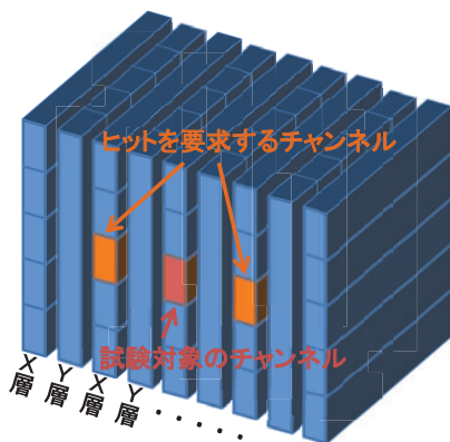
図 8.24 端のプレーン以外の宇宙線イベントの選択条件
