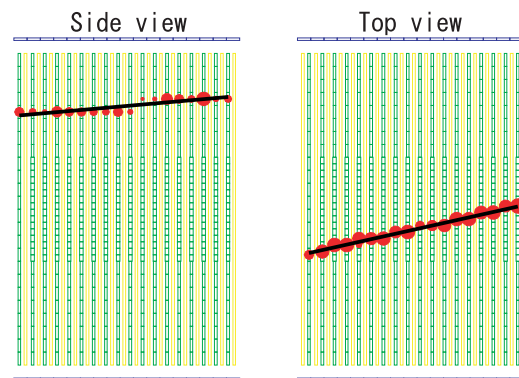
図 7.17 飛跡の最上流のヒットが最上流のプレーンがであるイベントの例
