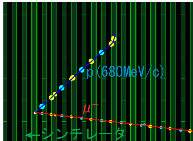
図 6.17 シミュレートされた Proton Module における CCQE イベント (左がビーム上流)
