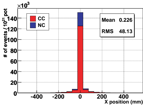
図 7.10 シミュレーションにより評価した、再構成された反応点 - 実際の反応点 (X 座標) 1 ビンは INGRID 型シンチレータの幅 (5cm)
