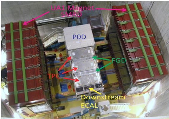
図 2.20 off-axis 検出器 (Magnet が開いている時)
