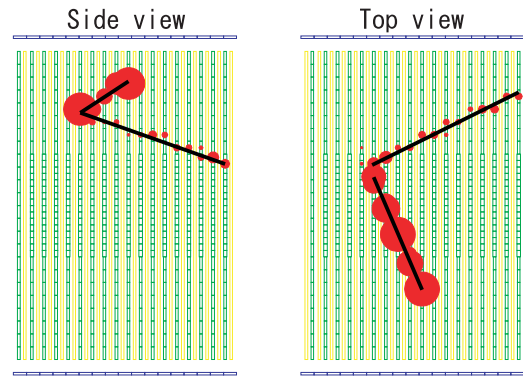
図 9.4 観測された CCQE 反応の候補 2 つの飛跡が観測でき、エネルギー損失が大きい飛跡が陽子、小さい飛跡がミュオンのものであると思われる。
