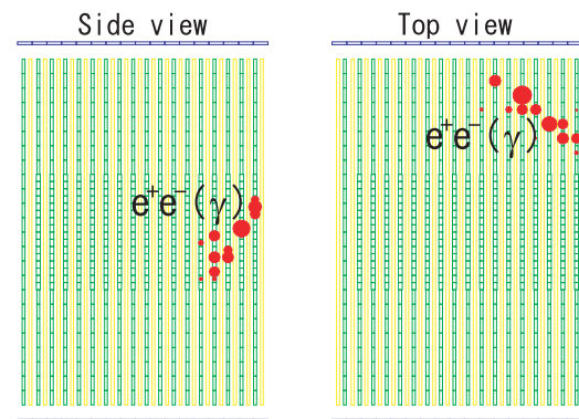
図 10.2 シミュレートされた外部から進入した \gamma が Proton Module で飛跡を残す電磁シャワーを起こしたイベントのイベントディスプレイ
