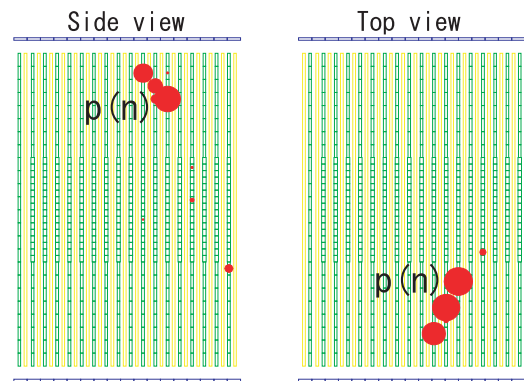
図 6.28 シミュレートされた壁での NC elastic 反応で放出された中性子が Proton Module で検出された例
