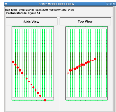
図 8.52 オンラインディスプレイで観測された宇宙線
