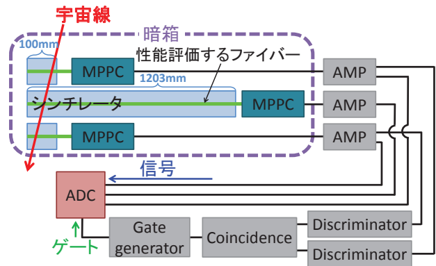
図 5.16 ファイバーの性能評価試験のセットアップ
