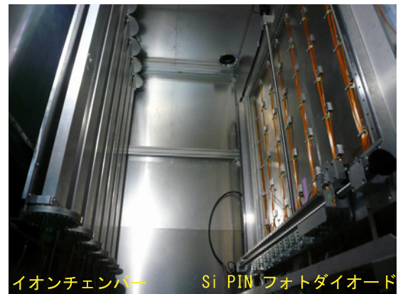
図 2.13 ミュオンモニター
