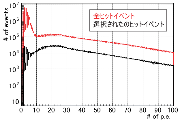
図 8.27 すべてのヒットイベントとイベント選択後のヒットイベントの光量分布
