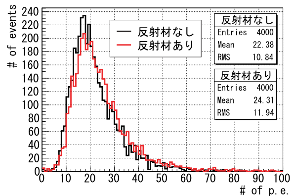
図 B.4 ファイバーの端面への反射材の塗布による光量分布の変化の典型例
