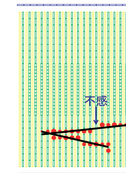
図 7.8 不感プレーンが 1 層あるイベントの例
