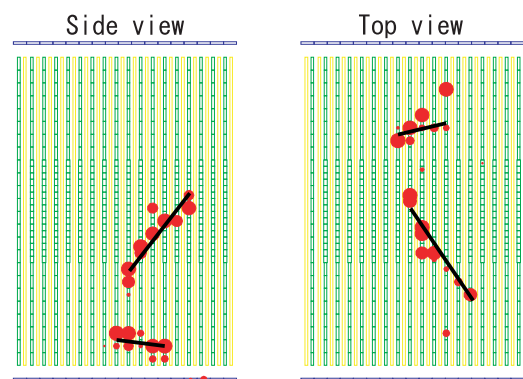
図 9.8 観測された NC\pi^0 反応の候補 離れた場所に 2 つの飛跡が観測されており、 \pi^0 の崩壊により生成された 2 つの \gamma だと思われる。
