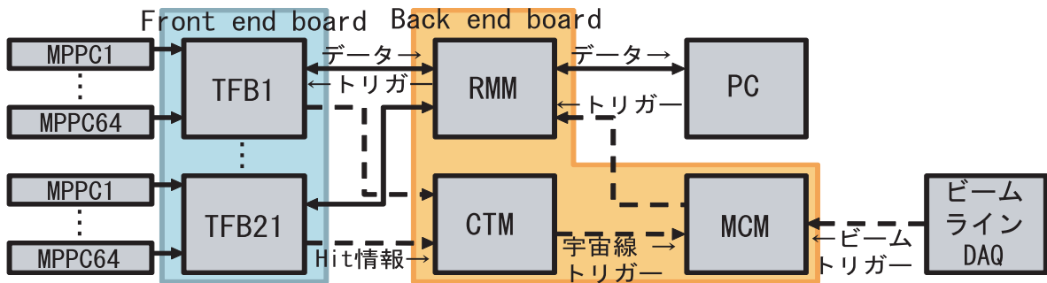
図 3.33 エレクトロニクス概要
