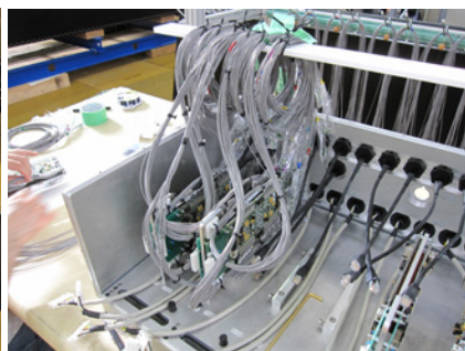
図 8.7 エレクトロニクスボックスへの TFB の取り付け
