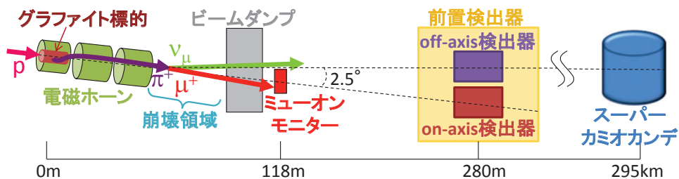
図 2.12 T2K 実験のビームライン
