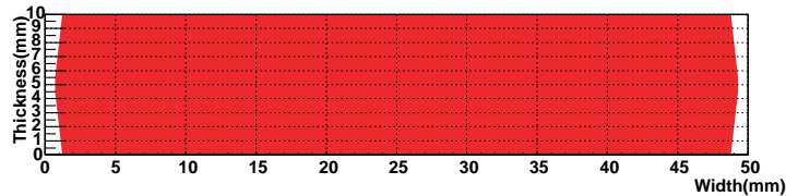
図 6.13 GEANT4 で再現した INGRID 型シンチレータの形 (赤の部分が有感領域、白の部分が不感領域)
