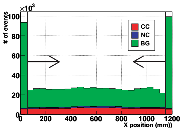
図 7.22 再構成された反応点の X 座標分布 (Veto プレーンによるカット後) 1 ピンは INGRID 型シンチレータの幅 (5cm)
