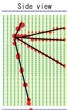
図 7.7 飛跡が 5 本あるイベントの飛跡再構成の例
