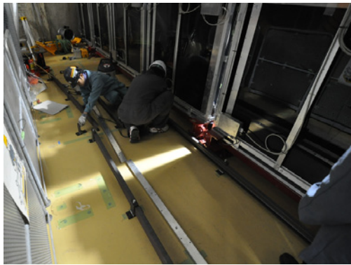
図 8.47 Proton Module 用のレールの設置
