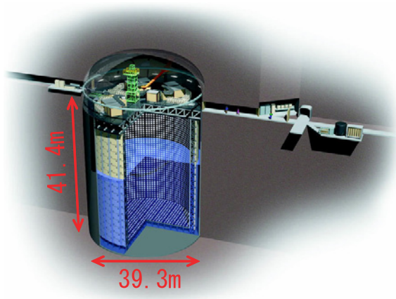
図 2.22 スーパーカミオカンデ概略図
