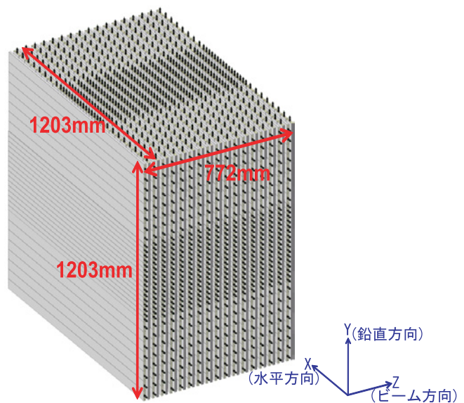
図 4.9 最上流のプレーンを除いたトラッキングプレーン
