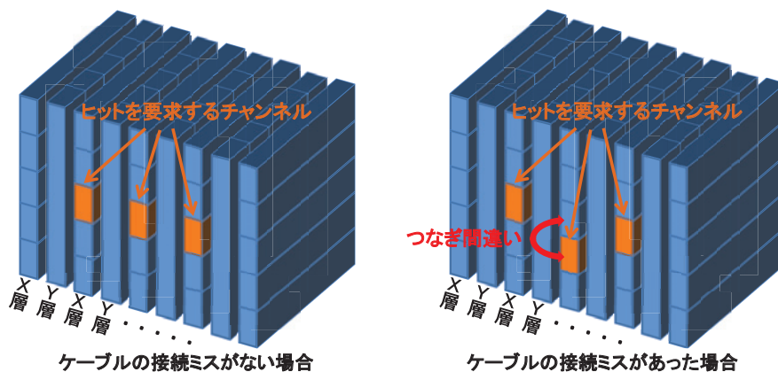
図 8.32 ケーブルミスがあった場合とない場合のイベント選択条件
