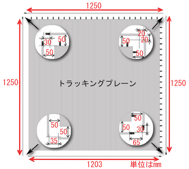
図 4.13 上流から見た Veto プレーンの位置
