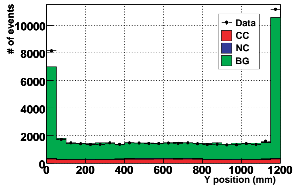
図 9.20 反応点の Y 座標分布 (Veto プレーンによるカット前)
