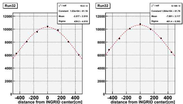
図 2.19 INGRID により求められたビームプロファイル (左が縦型モジュールにより求められた鉛直方向プロファイル、右が横型モジュールにより求められた水平方向プロファイル)
