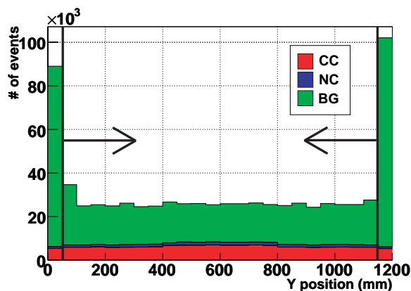
図 7.23 再構成された反応点の Y 座標分布 (Veto プレーンによるカット後) 1 ピンは INGRID 型シンチレータの幅 (5cm)
