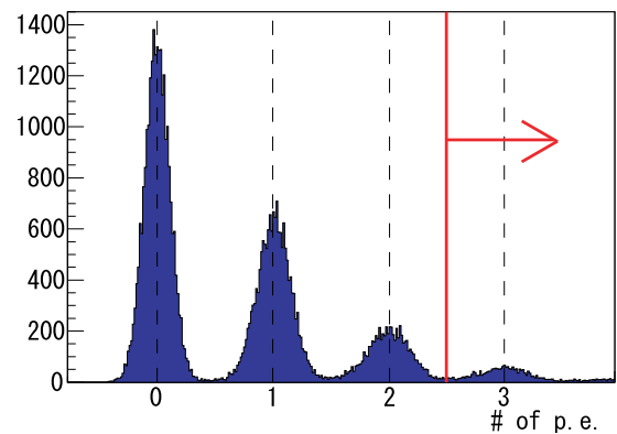
図 7.13 光量によるヒット選択
