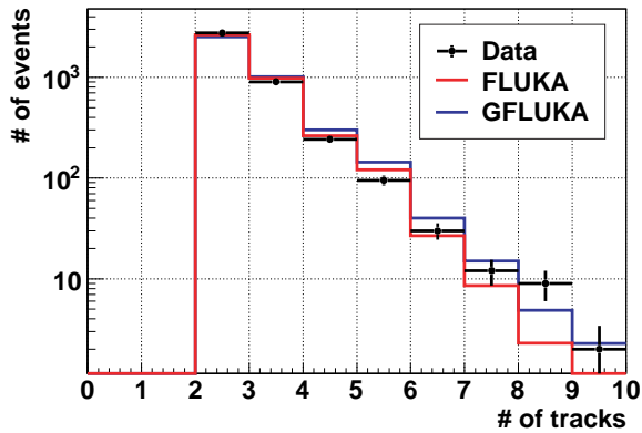
図 9.32 飛跡数分布の FLUKA, GFLUKA を用いた予測との比較 (反応数を規格化)
