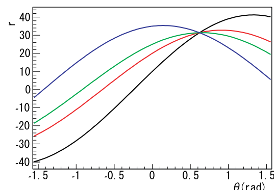
図 D.4 r\theta 平面における正弦曲線
