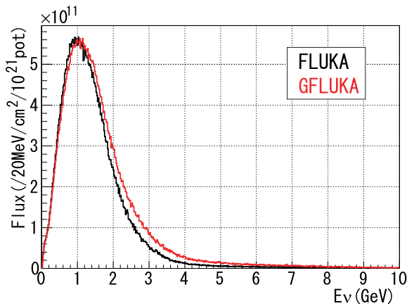
図 6.2 FLUKA と GFLUKA のハドロン生成モデルを用いた場合の Proton Module に入射するニュートリノのエネルギー分布
