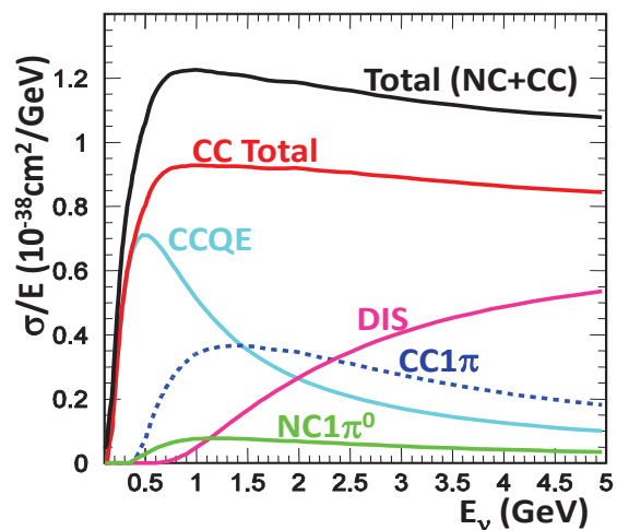
図 2.11 ニュートリノの反応断面積
