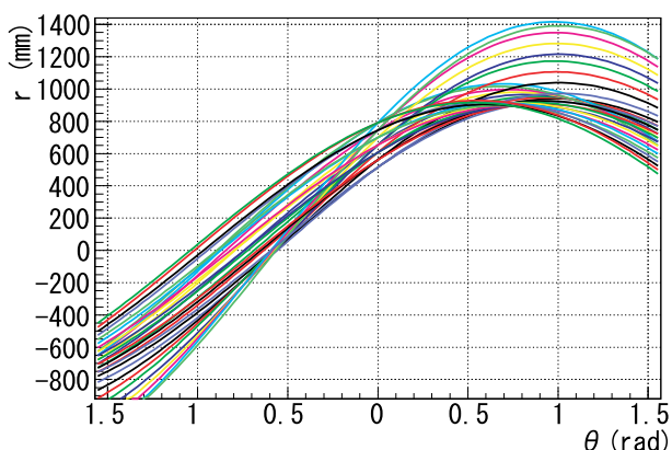
図 D.6 ヒットの位置をハフ変換した正弦曲線
