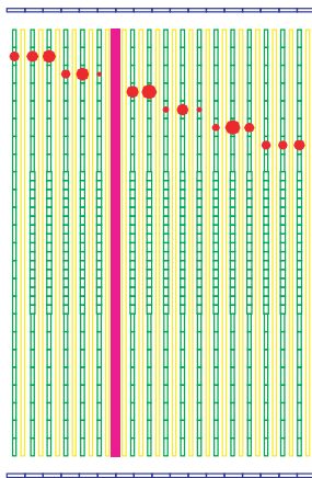
図 8.40 評価するプレーンのヒット情報を隠す
