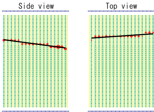
図 9.3 観測された外部から入射した荷電粒子によるイベントの候補 光量が低いことから、ミュオンの飛跡であると思われる。
