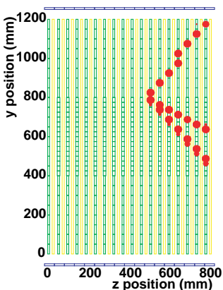
図 D.5 ヒットがあったシンチレータの 2 次元位置
