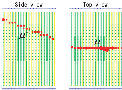
図 6.25 シミュレートされた壁での CCQE 反応で生成されたミュオンが Proton Module の最上流のトラッキングプレーンで検出された例
