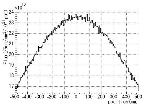
図 6.3 Proton Module の移動可能範囲におけるニュートリノフラックス
