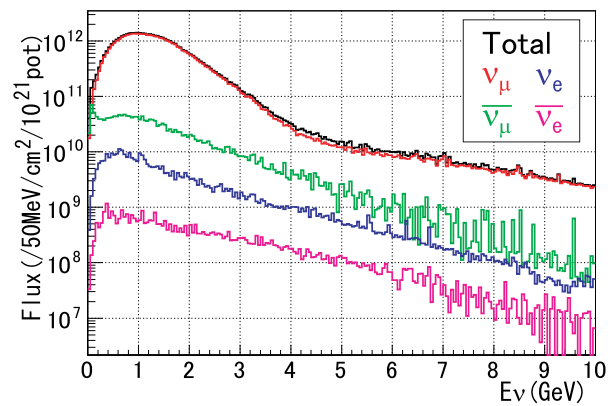
図 6.4 各フレーバーのニュートリノのエネルギー分布
