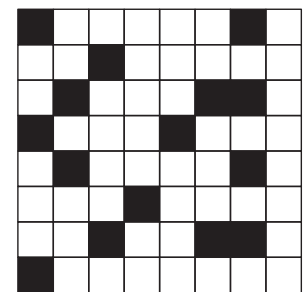
図 D.9 ライフゲームの例
