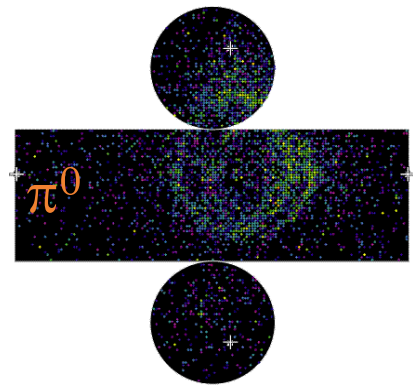
図 2.26 スーパーカミオカンデにおける \pi^0 イベント (シミュレーション)
