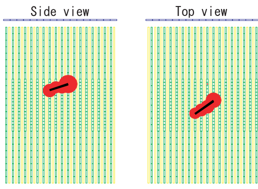
図 9.7 観測された NC Elastic 反応の候補 1 つの飛跡が観測でき、エネルギー損失が大きいことから陽子と思われる。
