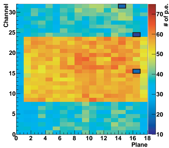
図 8.28 X 層の各シンチレータでの宇宙線イベントの平均光量 (黒い四角で囲まれたチャンネルの光量が低い)
