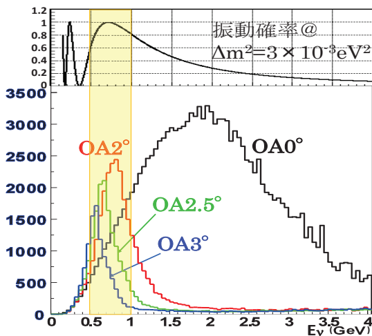
図 2.10 ニュートリノ振動確率 (上) と off-axis 法によるニュートリノエネルギー分布 (下)
