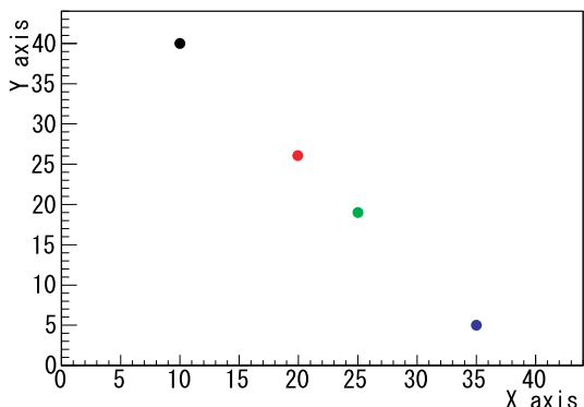
図 D.3 xy 平面において直線上にある点
