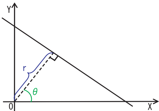
図 D.1 xy 平面における r と \theta
