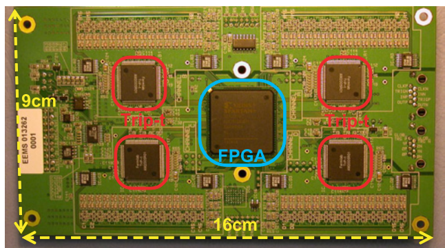
図 3.31 TFB の裏側
