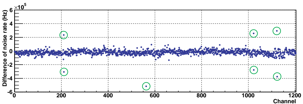
図 8.17 組立前と組立後のノイズレートの測定値の差 (緑色の丸で囲まれた点が差が激しいチャンネル)
