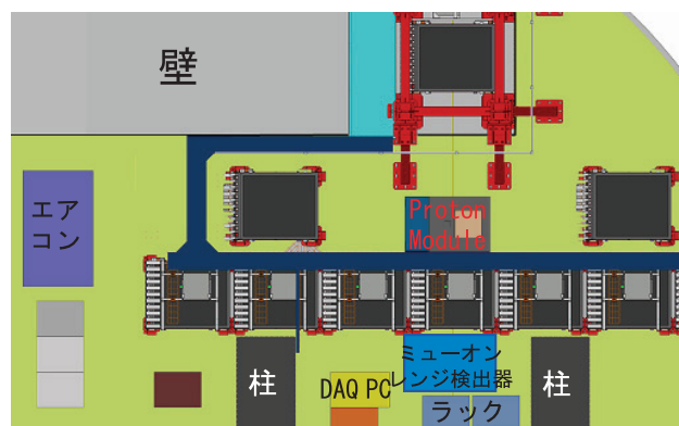
図 F.4 ミュオンレンジ検出器の設置
