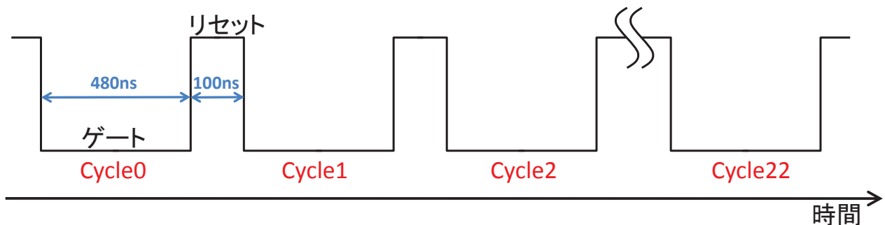
図 3.34 ゲートとリセットの時間
