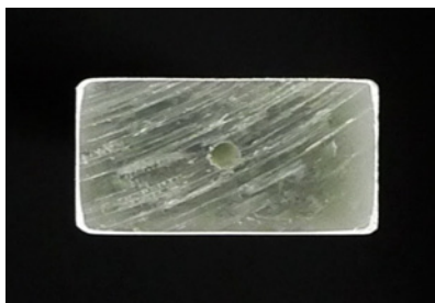
図 6.14 SciBar 型シンチレータの断面 (周りの白い部分が反射材)
