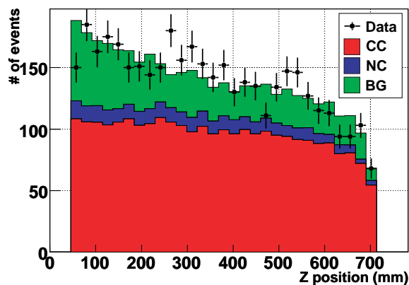
図 9.29 反応点の Z 座標分布
