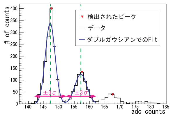
図 5.5 ピークから \pm 3\sigma の範囲で積分
