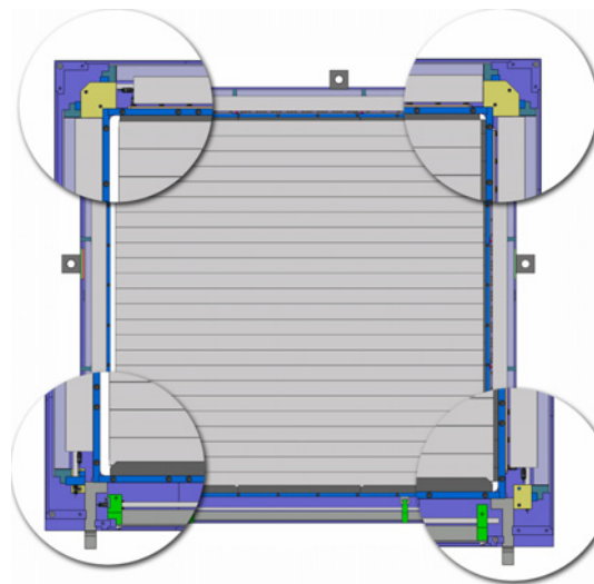
図 F.2 増設する Veto 用シンチレータの位置
