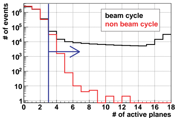
図 9.13 アクティブプレーン数の分布
