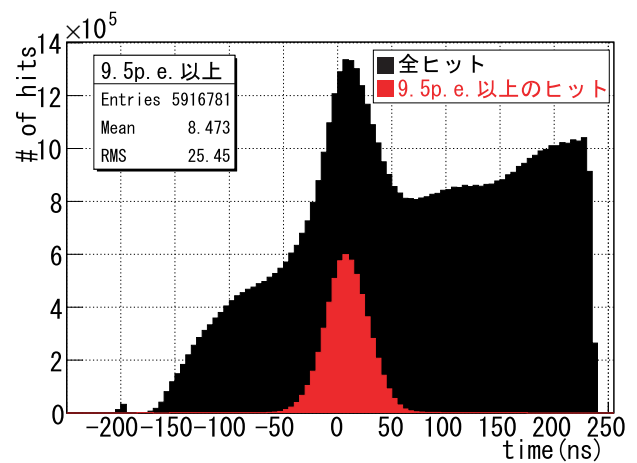
図 9.12 ビームサイクルにおいて観測されたヒットイベントのヒット時間と期待されるヒット時間範囲の中心値の差
