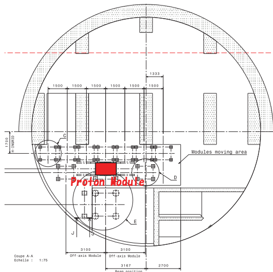
図 6.23 前置検出器ホールの形と Proton Module の設置位置 (下がビーム上流)
