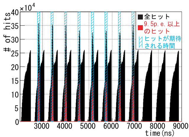
図 9.11 4 番目から 15 番目までのサイクルにおいて観測されたヒットイベントのヒット時間分布 (それぞれのピークがサイクルに対応する)
