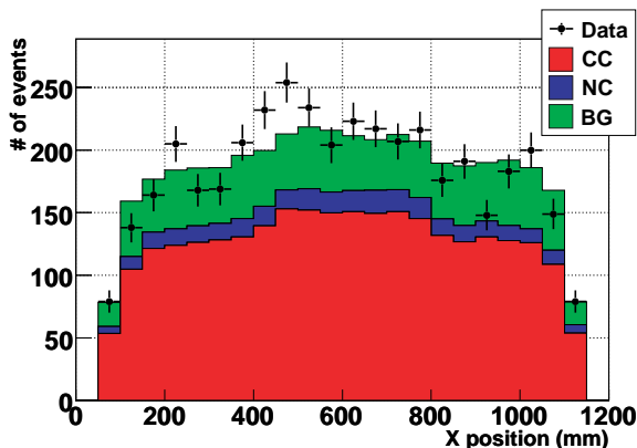
図 9.27 反応点の X 座標分布
