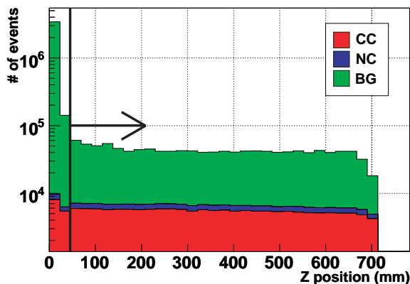
図 7.16 再構成された反応点の Z 座標分布 1 ビンはトラッキングプレーン間の距離 (2.3cm)
