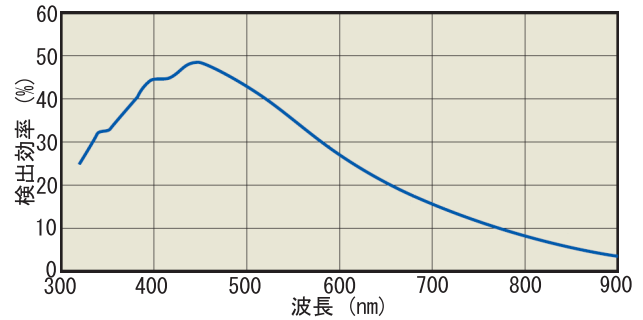
図 3.17 MPPC(S10362-13-050C) の検出効率の波長依存性
