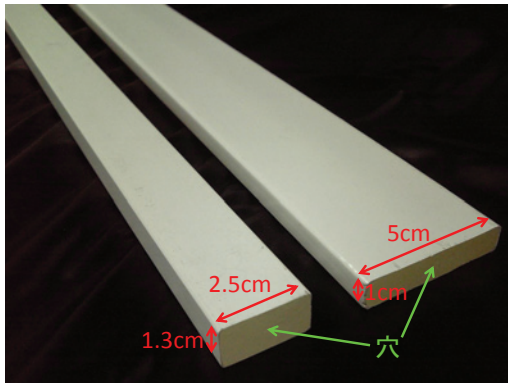
図 3.13 左が SciBar 型シンチレータ、右が INGRID 型シンチレータ
