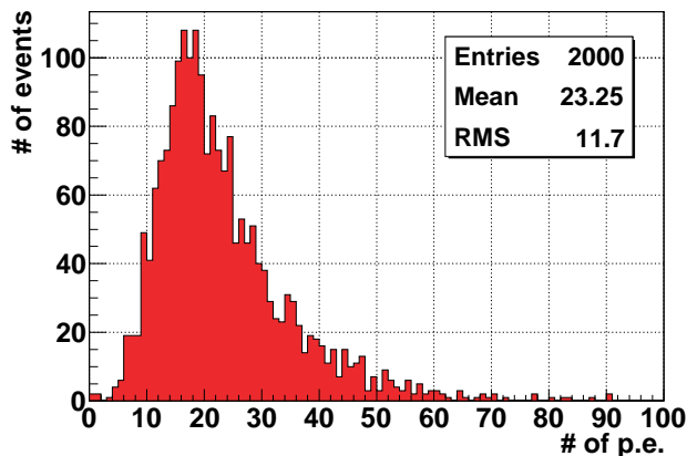
図 5.17 1 本のファイバー試験での典型的な光量分布
