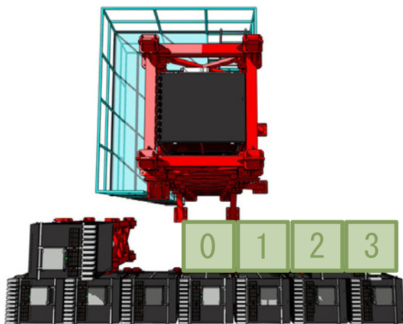
図 6.5 Proton Module の設置位置 (上から)
