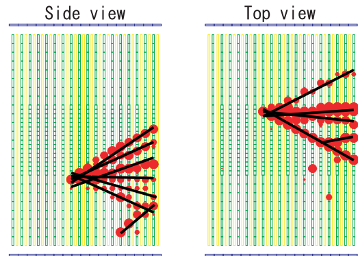
図 9.6 観測された DIS 反応の候補 ニュートリノ反応と思われる点から多数の粒子が放出されている。
