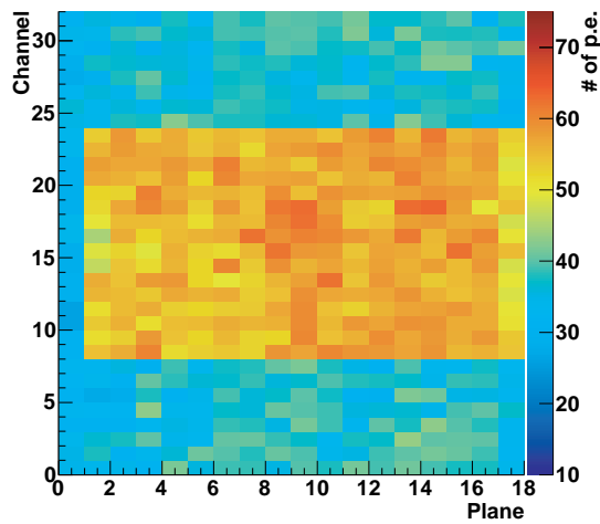
図 8.30 修繕後の X 層の各シンチレータでの宇宙線イベントの平均光量
