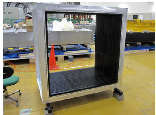
図 8.1 Proton Module 用フレーム 内側には溝の刻まれた板が付いている
