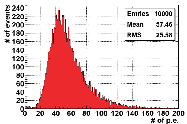
図 5.13 SciBar 型シンチレータの典型的な光量分布
