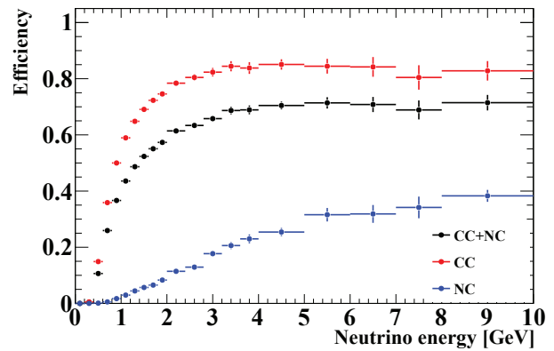
図 3.8 INGRID の検出効率 [23] 。0.4GeV 未満のニュートリノの検出効率は 0% である。
