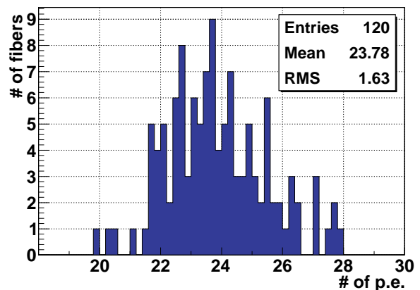
図 5.18 120 本のファイバーからの平均光量分布
