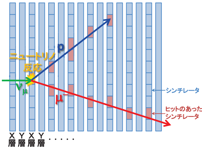
図 3.9 ニュートリノ検出の概念図
