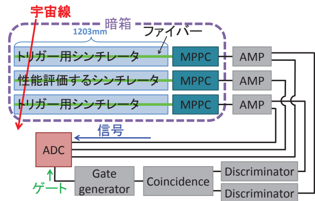
図 5.11 シンチレータの性能評価試験のセットアップ
