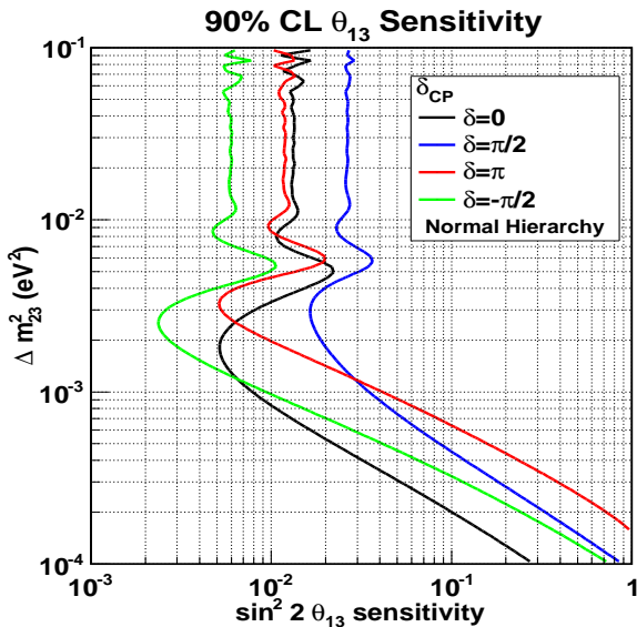
図 2.2 T2K 実験の \theta_{13} への感度 (90% C.L.) \sin^2 2\theta_{12} = 0.8704 , \sin^2 2\theta_{23} = 1.0 , \Delta m_{12}^2 = 7.6 \times 10^{-5} \text{eV}^2 , 5 \times 10^{21} \text{POT} , 標準階層, 系統誤差=10% のとき
