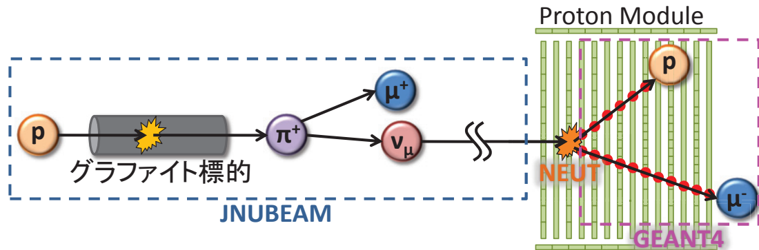
図 6.1 Proton Module におけるモンテカルロ・シミュレーションの概念図
