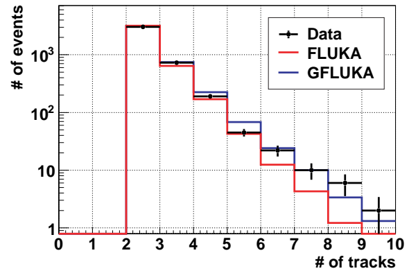
図 9.33 同じ反応点からの飛跡数分布の FLUKA, GFLUKA を用いた予測との比較 (反応数を規格化)
