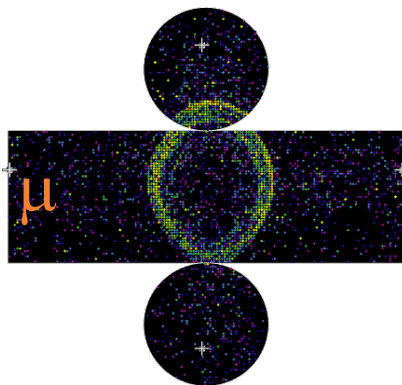
図 2.24 スーパーカミオカンデにおけるミュオンイベント (シミュレーション)
