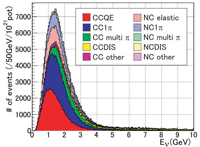
図 6.8 Proton Module において相互作用をしたニュートリノのエネルギー分布と反応モード
