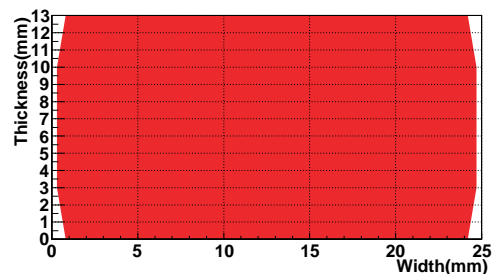
図 6.15 GEANT4 で再現した SciBar 型シンチレータの形 (赤の部分が有感領域、白の部分が不感領域)
