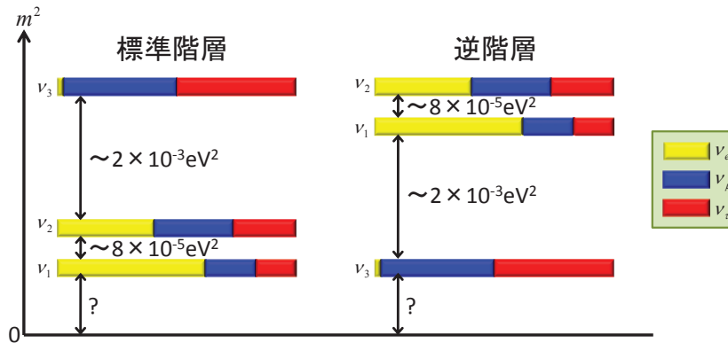
図 1.5 質量階層
