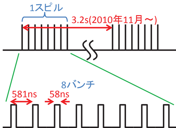
図 2.6 T2K 実験における陽子ビームの時間構造
