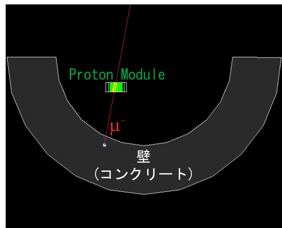
図 6.24 GEANT4 において前置検出器ホールの壁におけるニュートリノ反応からの二次粒子が Proton Module に入射したイベントの例 (下がビーム上流)
