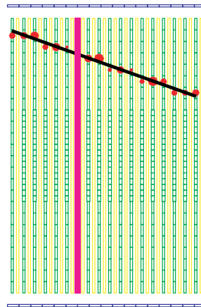
図 8.41 ヒット情報を隠したままで飛跡を再構成
