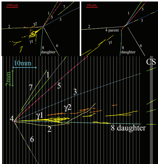
図 1.3 OPERA 実験において初観測されたタウニュートリノ出現イベントの候補 8 番の飛跡がタウニュートリノ候補の崩壊による娘粒子とされている。
