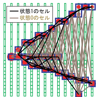
図 7.3 ステップ 1 におけるセルの状態
