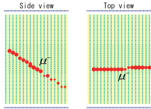
図 6.26 シミュレートされた壁での CCQE 反応で生成されたミュオンが Proton Module の最上流のトラッキングプレーンの隙間を抜けた例
