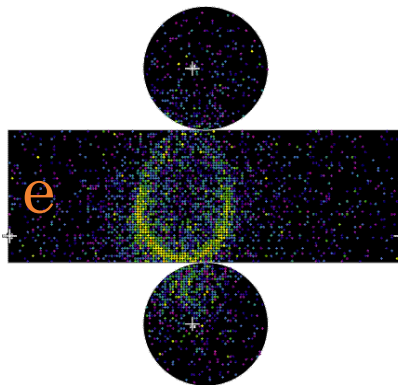
図 2.25 スーパーカミオカンデにおける電子イベント (シミュレーション)
