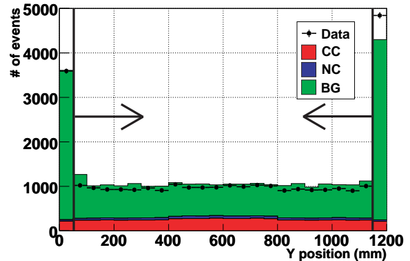
図 9.22 反応点の Y 座標分布 (Veto プレーンによるカット後)
