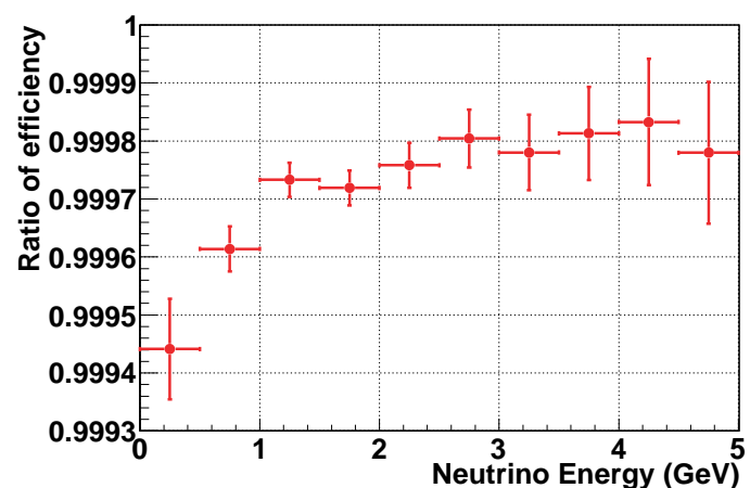
図 8.55 全てのチャンネルが有感の場合と 1 つ不感チャンネルがある場合の検出効率の比
