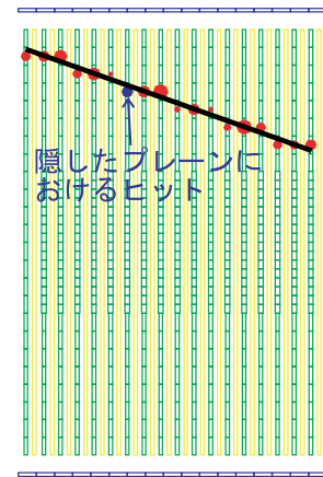
図 8.42 飛跡が評価するプレーンを突き抜けていれば評価するプレーンにヒットがあるか確認
