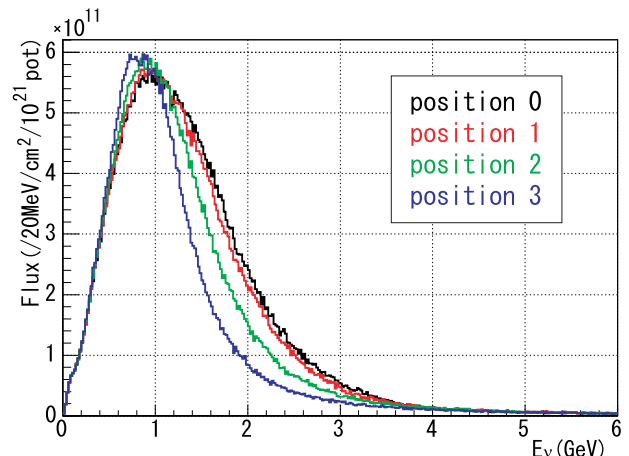
図 6.6 各設置位置におけるニュートリノフラックスのエネルギー分布
