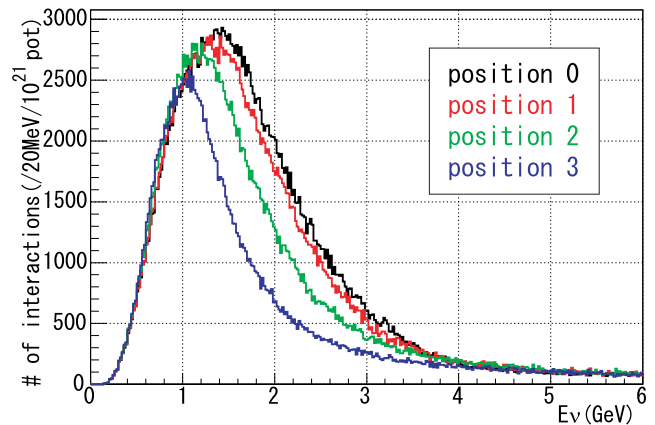
図 6.10 各設置位置において反応したニュートリノのエネルギー分布
