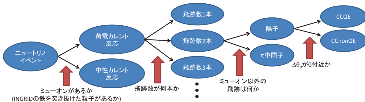
図 10.5 CCQE 反応の選択のための解析の流れ
