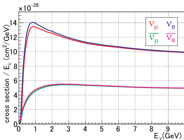
図 6.7 NEUT におけるニュートリノのシンチレータ (CH) との反応断面積
