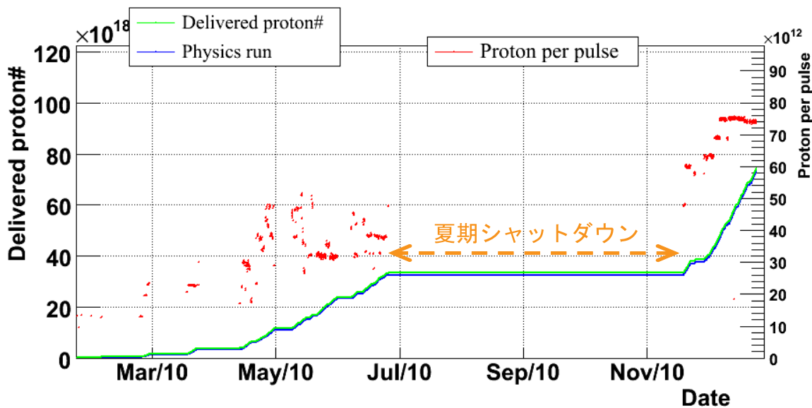
図 A.5 累積 POT 数とパルスあたりの POT 数の推移
