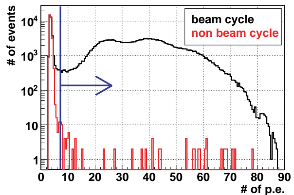
図 9.14 アクティブプレーン数が 3 以上のイベントのアクティブプレーンあたりの光量分布
