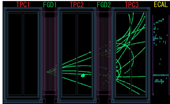
図 2.21 off-axis 検出器のイベントディスプレイ
