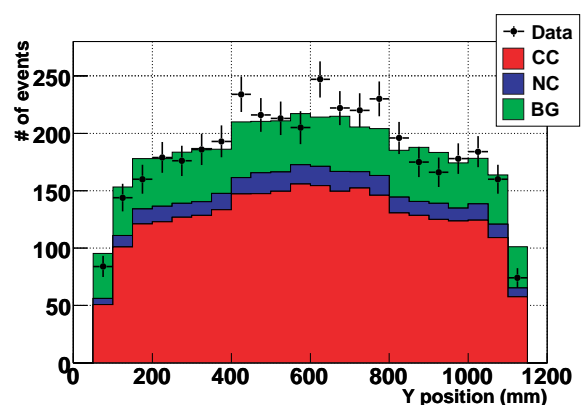
図 9.28 反応点の Y 座標分布
