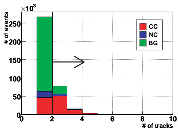
図 7.25 飛跡数分布
