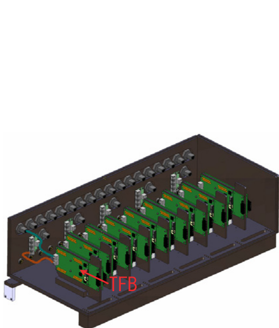
図 4.19 エレクトロニクスボックス
