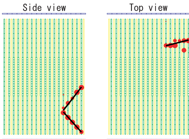
図 9.1 Proton Module における最初のニュートリノイベントのイベントディスプレイ
