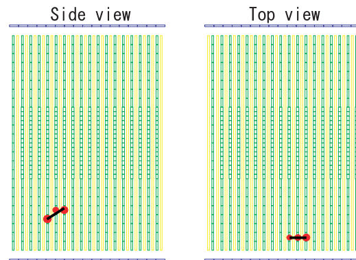
図 7.15 X 層と Y 層の飛跡が合致しないイベントの例
