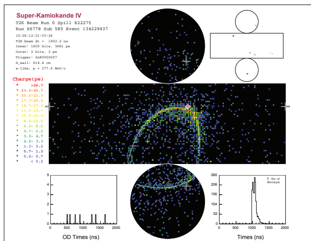
図 A.7 スーパーカミオカンデにおいて観測された電子ニュートリノ出現イベントの候補
