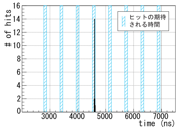
図 9.2 Proton Module における最初のニュートリノイベントのヒット時間分布
