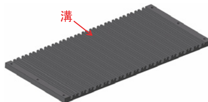
図 4.15 シンチレータ固定のための溝が刻まれた板
