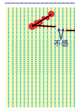
図 7.9 不感プレーンが 2 層続いたイベントの例
