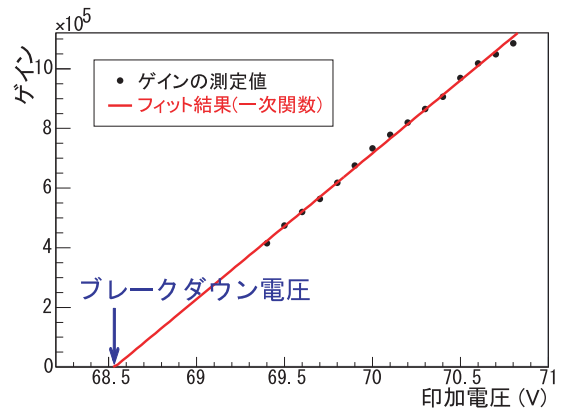
図 5.6 ブレークダウン電圧の算出方法
