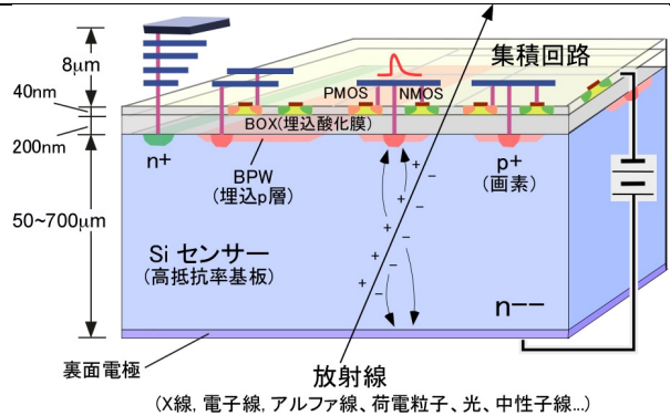
図 2 SOI 量子イメージングセンサー構造
