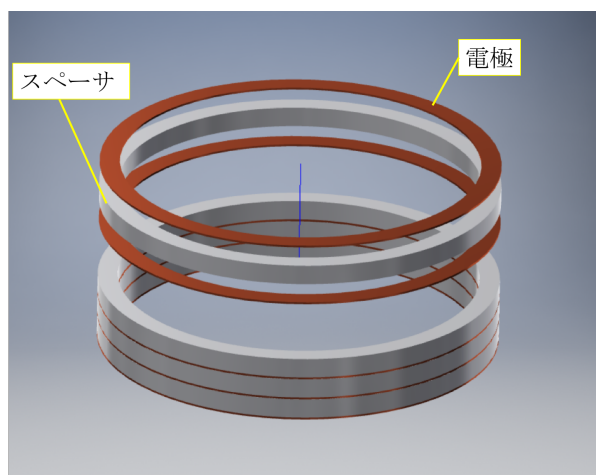
図 4.3 リング型フィールドケージの概念図
