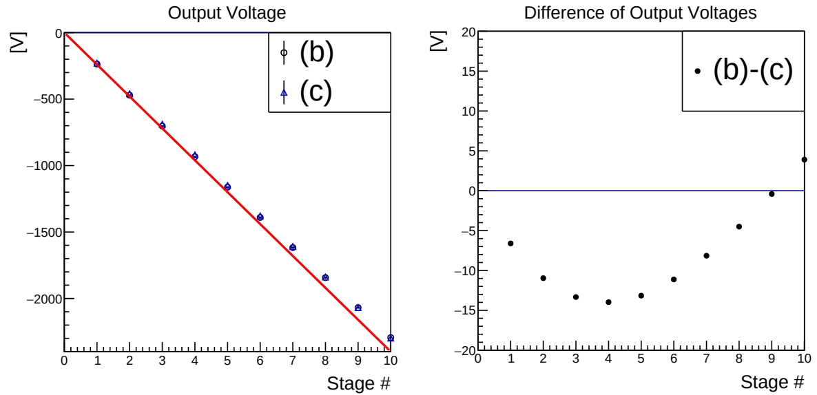
図 5.5 (b) の方法と (c) の方法での各段の出力電圧 (左) とその差 (右) のシミュレーション。赤線は理想的な場合の出力 2NU 。
