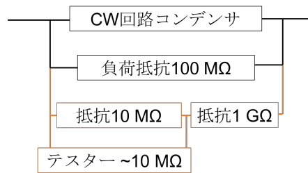
図 5.8 CW 回路各段の電位差の測定方法。色をつけた部分が測定系。
