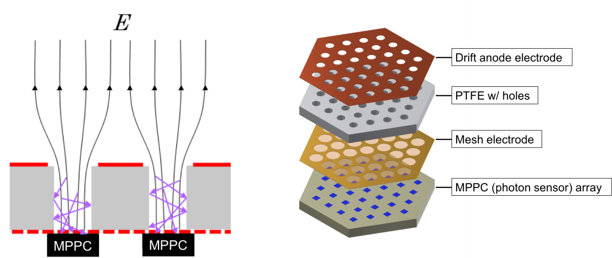
図 2.3 ELCC 概念図。1 セルの断面図 (左) と層構造の全体 (右)。
