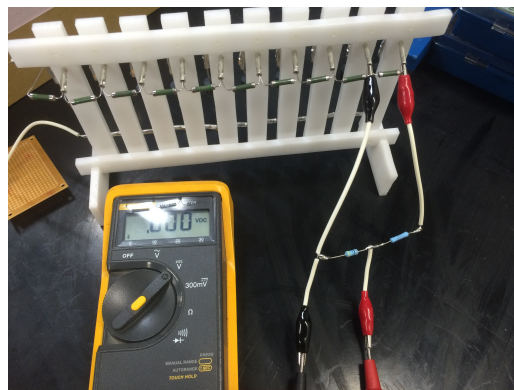
図 5.6 リード型試作回路。コンデンサとダイオードによる CW 回路本体の面 (左) と負荷抵抗の面 (右)
