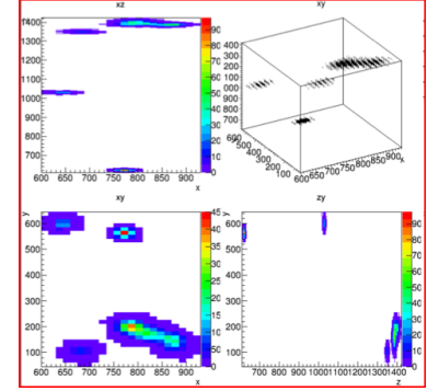
図 2.2 各反応について AXEL 検出器で得られる飛跡のシミュレーション。各反応につき右上が三次元飛跡でその他が平面への射影。[19]
