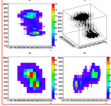
図 2.2 各反応について AXEL 検出器で得られる飛跡のシミュレーション。各反応につき右上が三次元飛跡でその他が平面への射影。[19]
