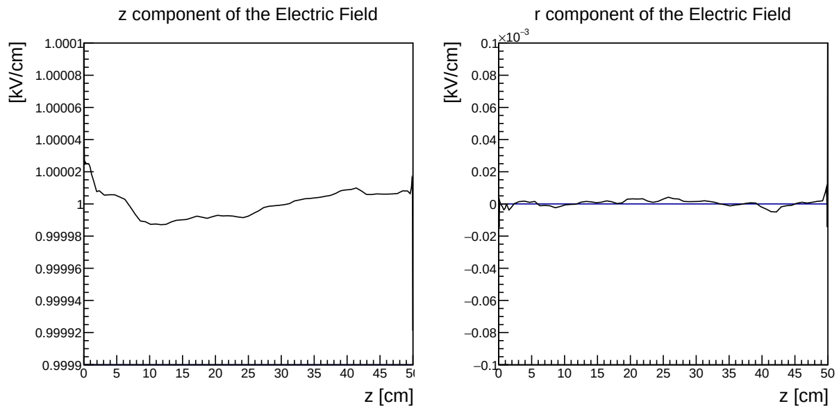
図 4.18 帯状電極埋め込み型フィールドケージの中心軸上での電場の z 成分と r 成分
